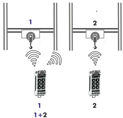
Fonctionnement deux différentes grues portiques avec deux commandes différentes
